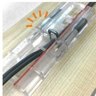
細いケーブルの場合
